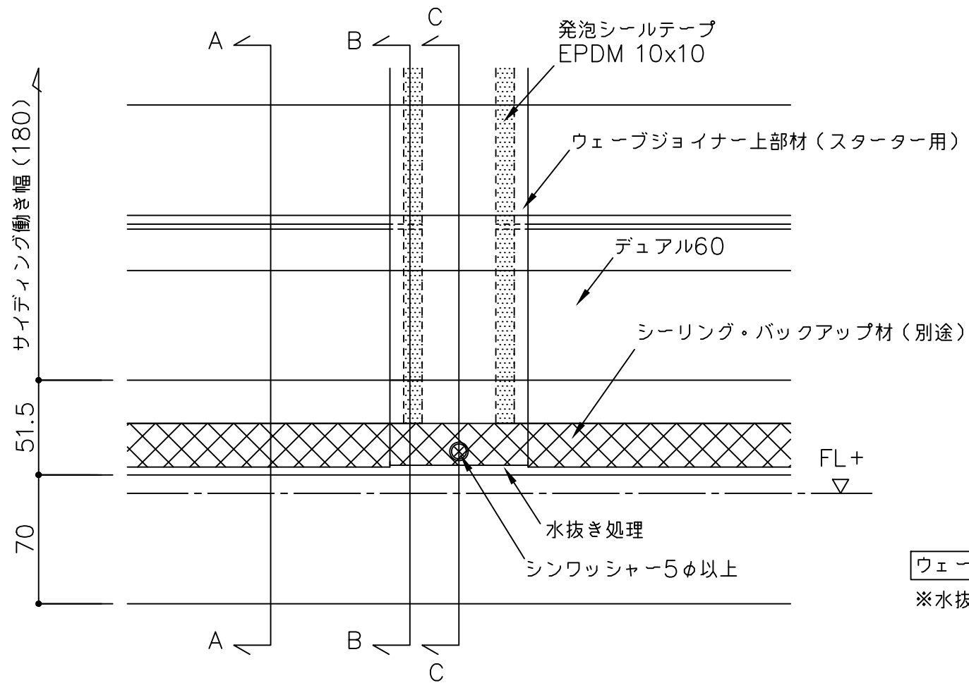
B部断面図
