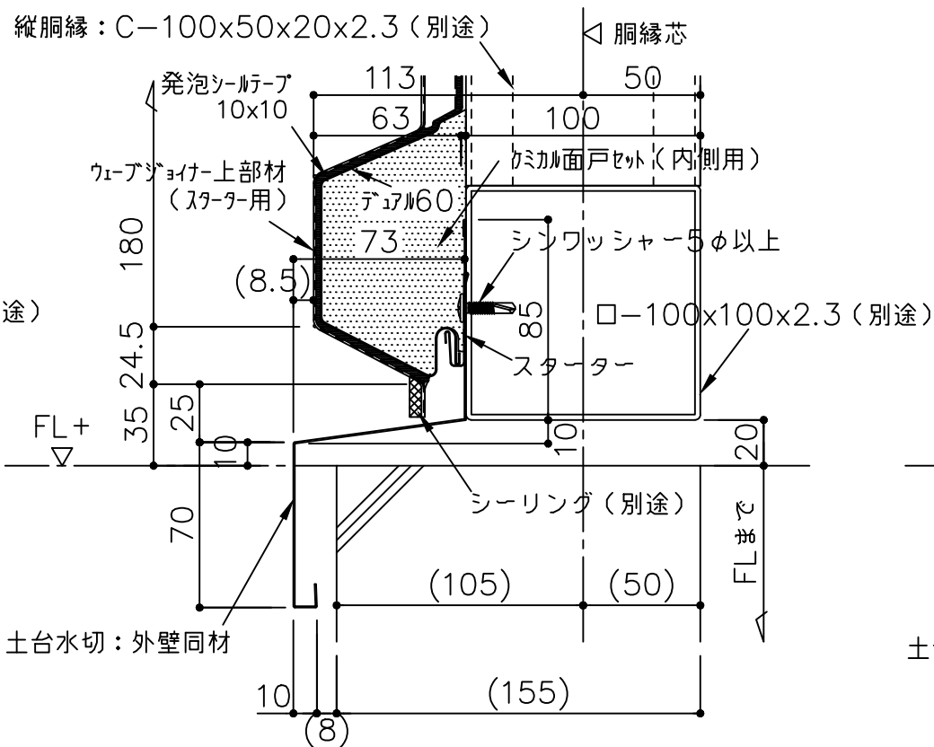
B部断面図
