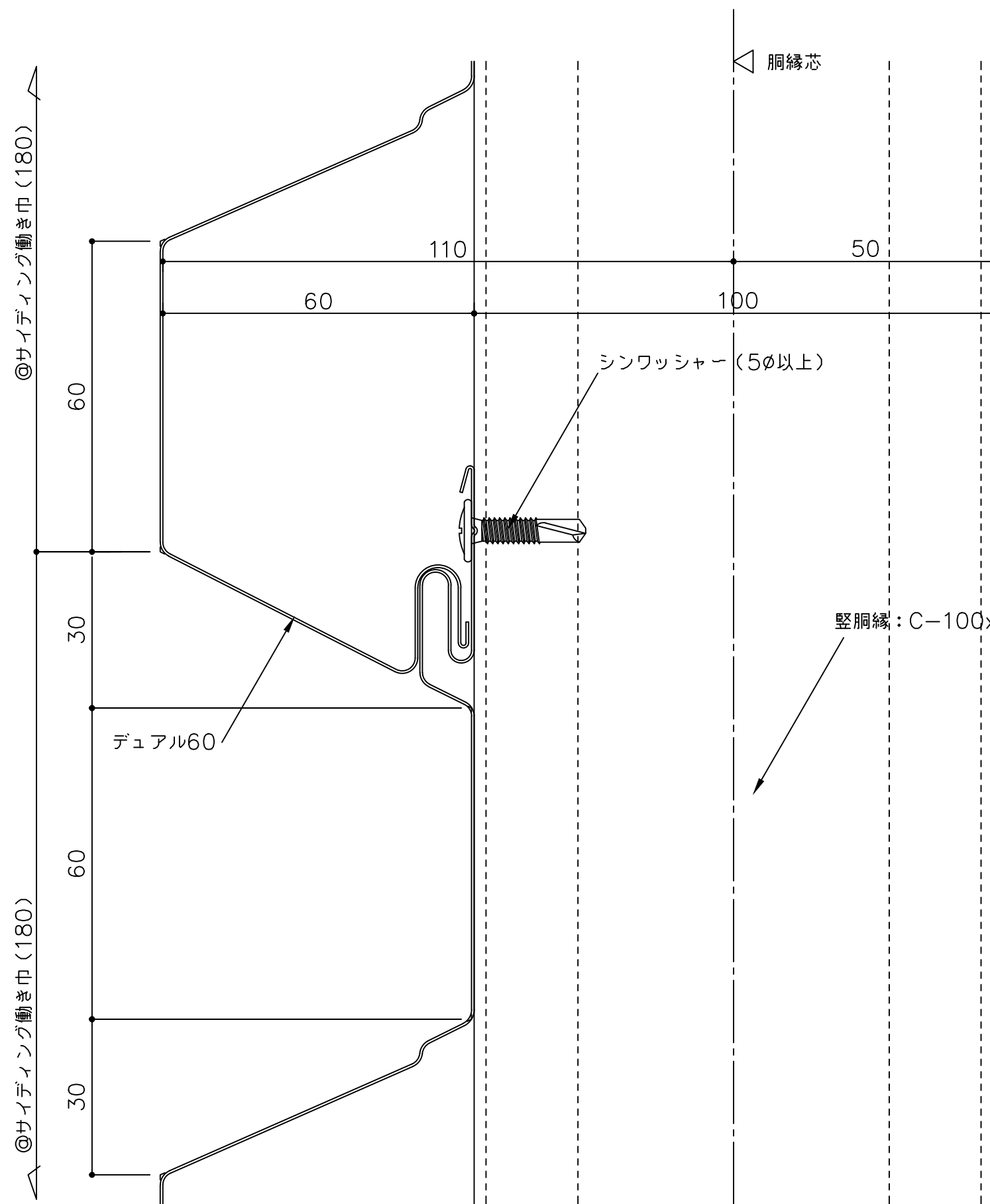
かん合部詳細図 1:1
