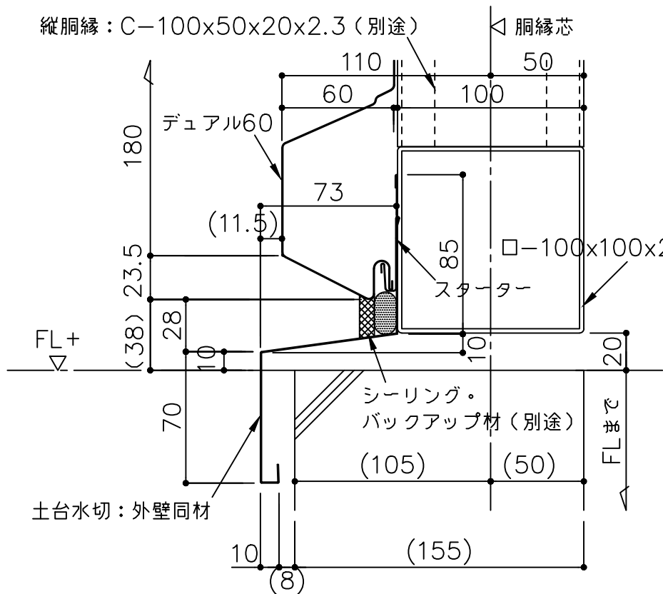
A部断面図
