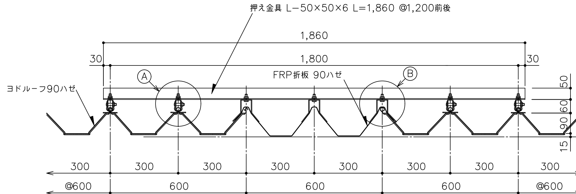
断面詳細図 1/10
