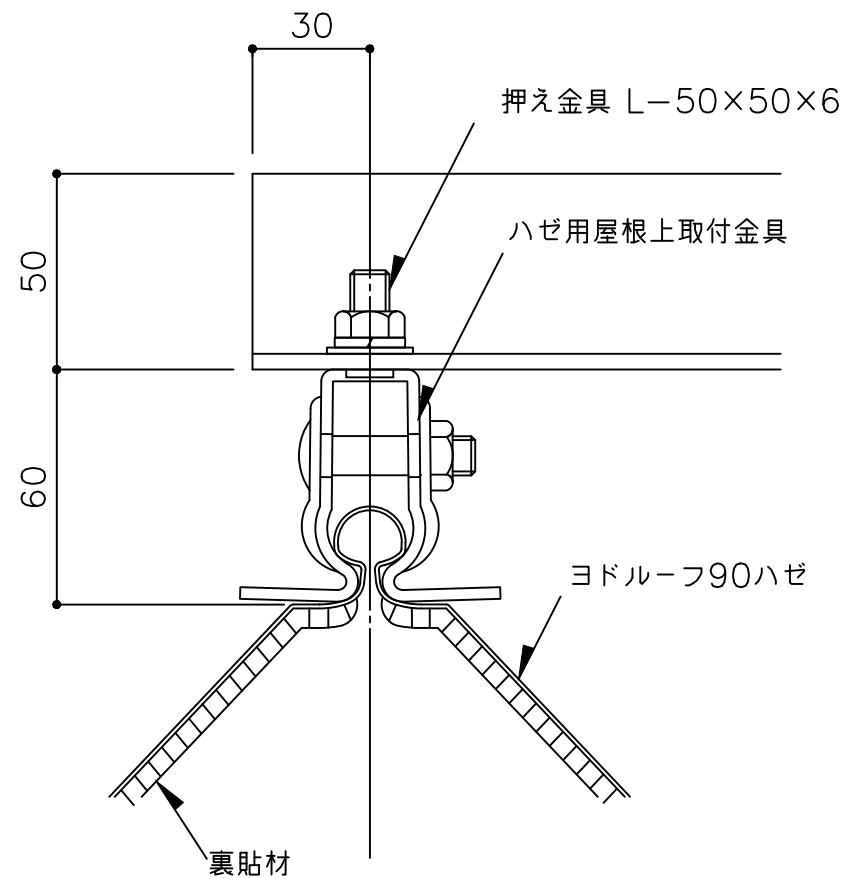
A 詳細図 1/2
