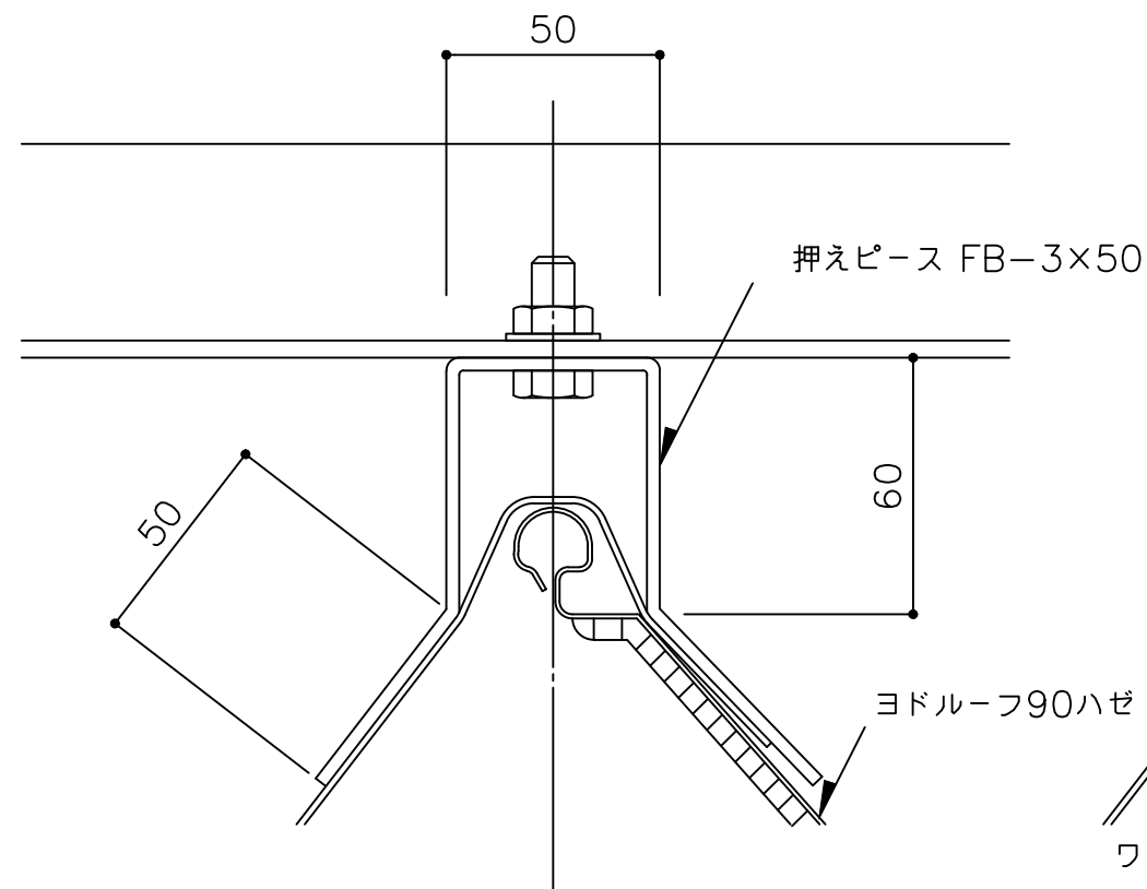
B 詳細図 1/2
