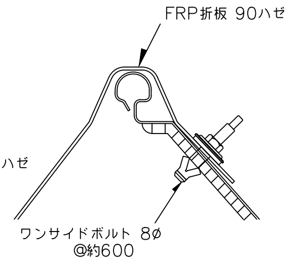
B' 中間部詳細図 1/2
