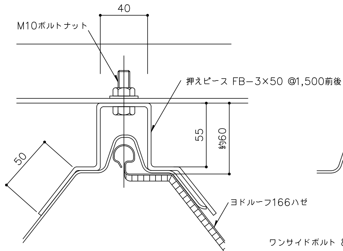
B 詳細図 1/2
